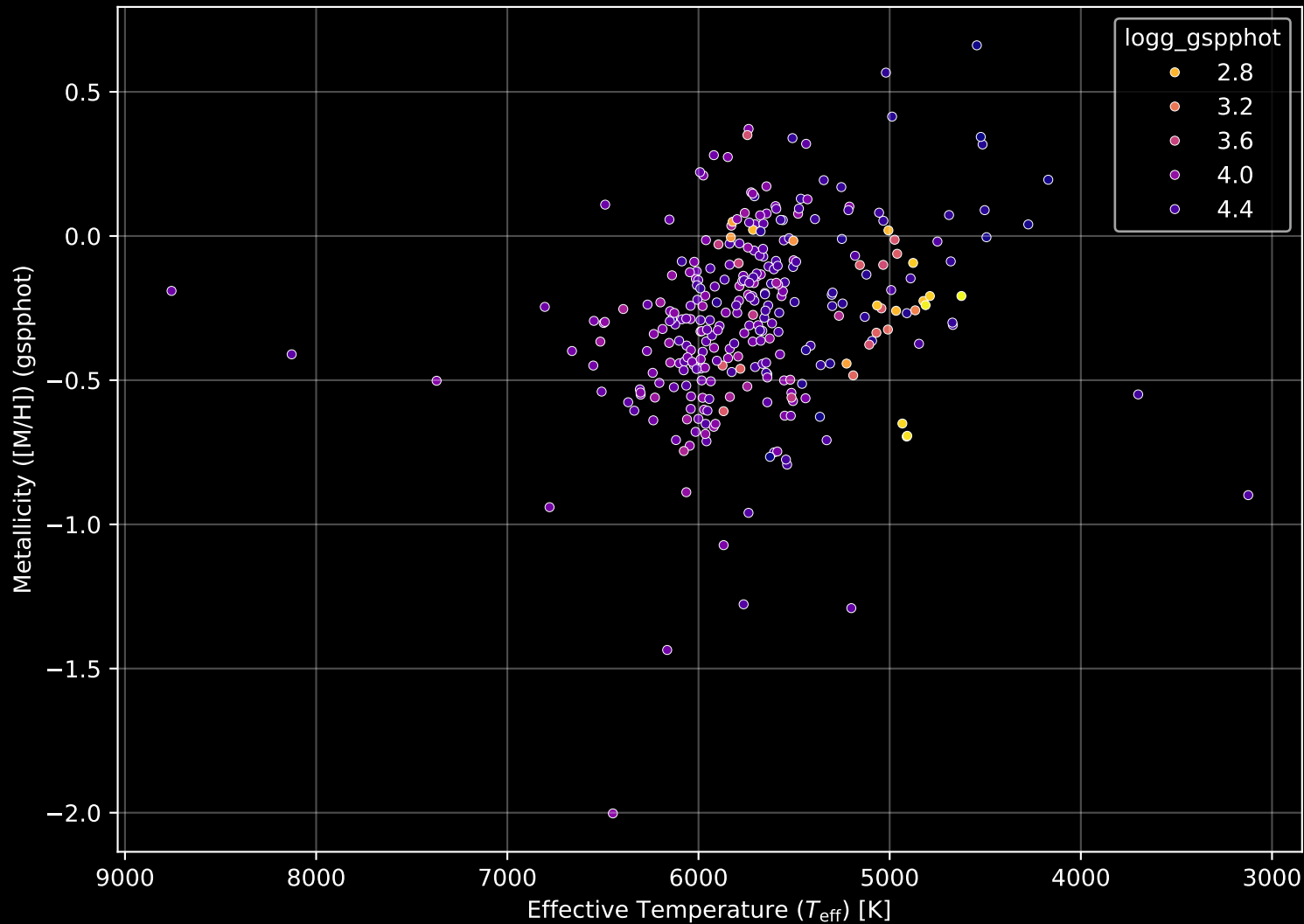
GALAH DR4 Field: [451] Stellar Population Parameters (n= 302)
