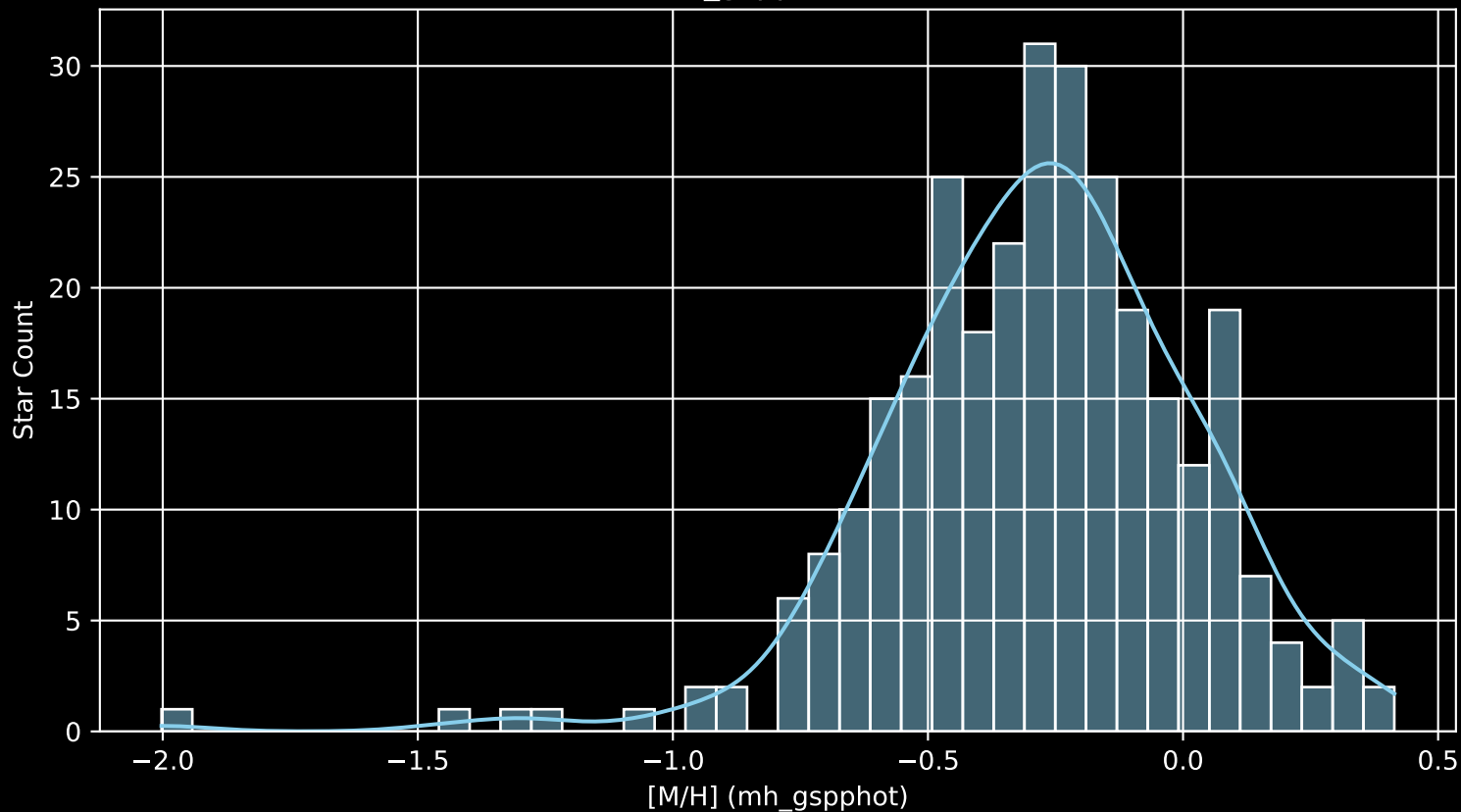
GALAH DR4 Field: [451] [M/H] (mh_gspphot) (n= 300)
