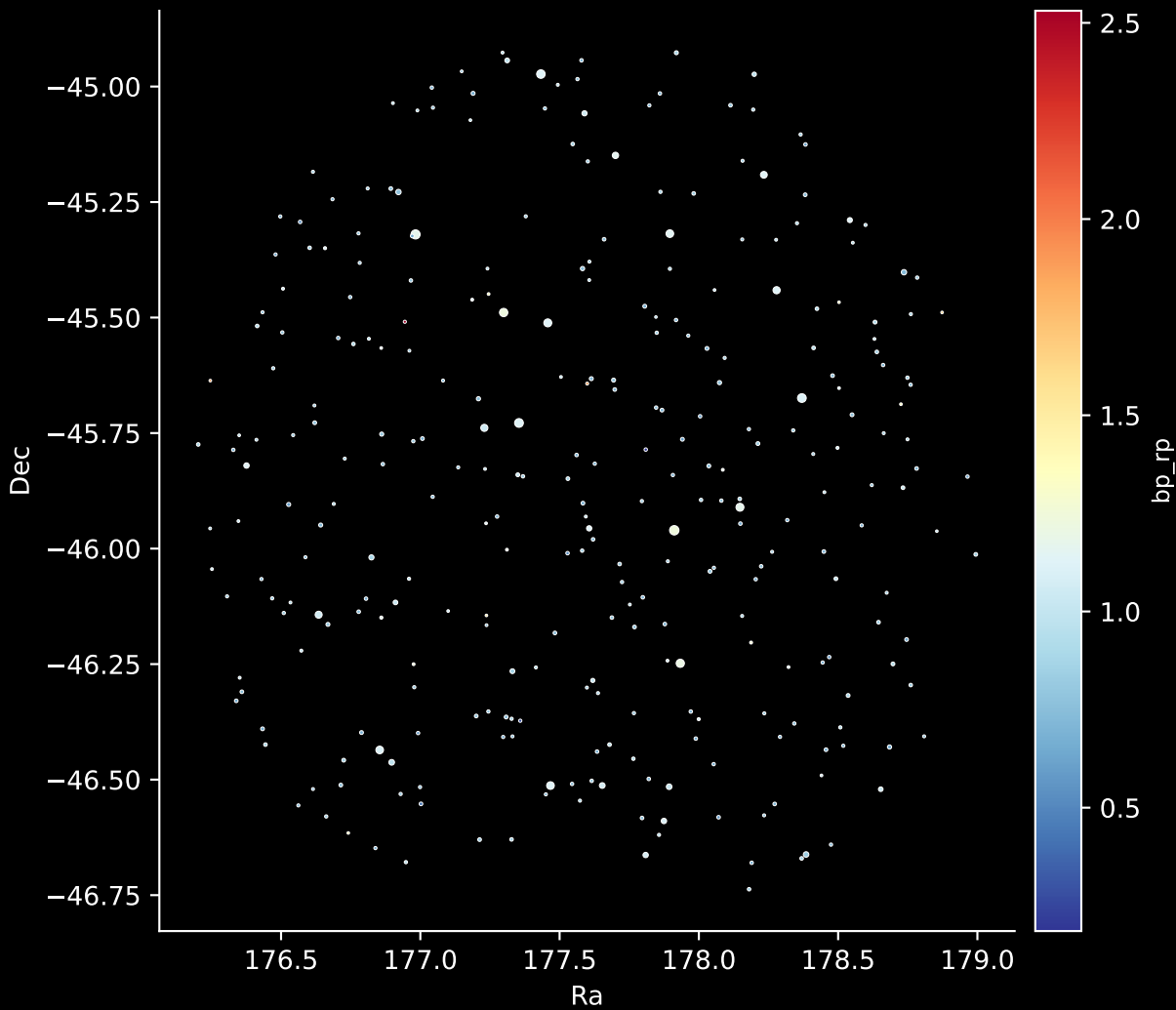
GALAH DR4 Field: [451] Stars: 302
