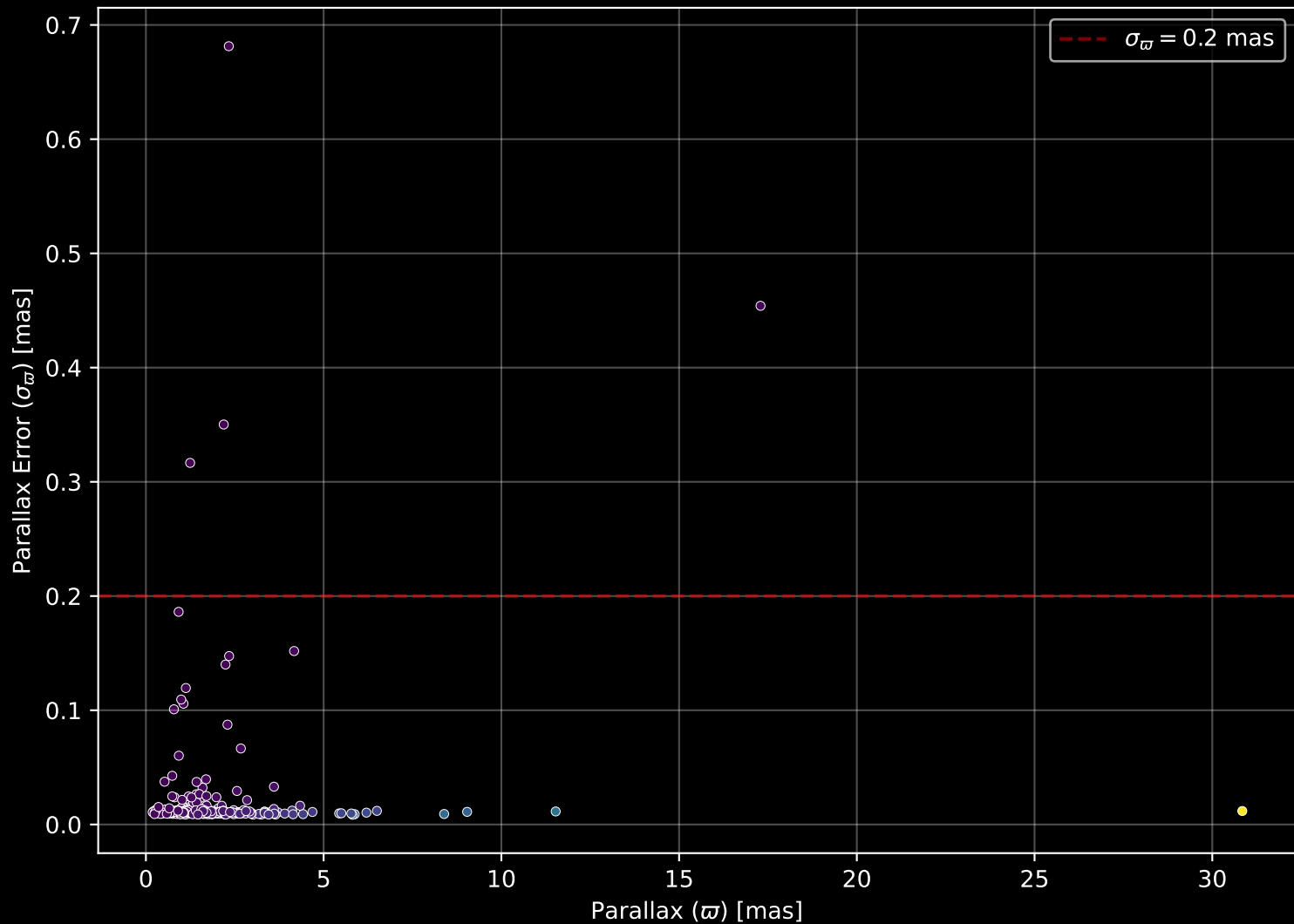
GALAH DR4 Field: [451] Parallax Quality (n= 302)
